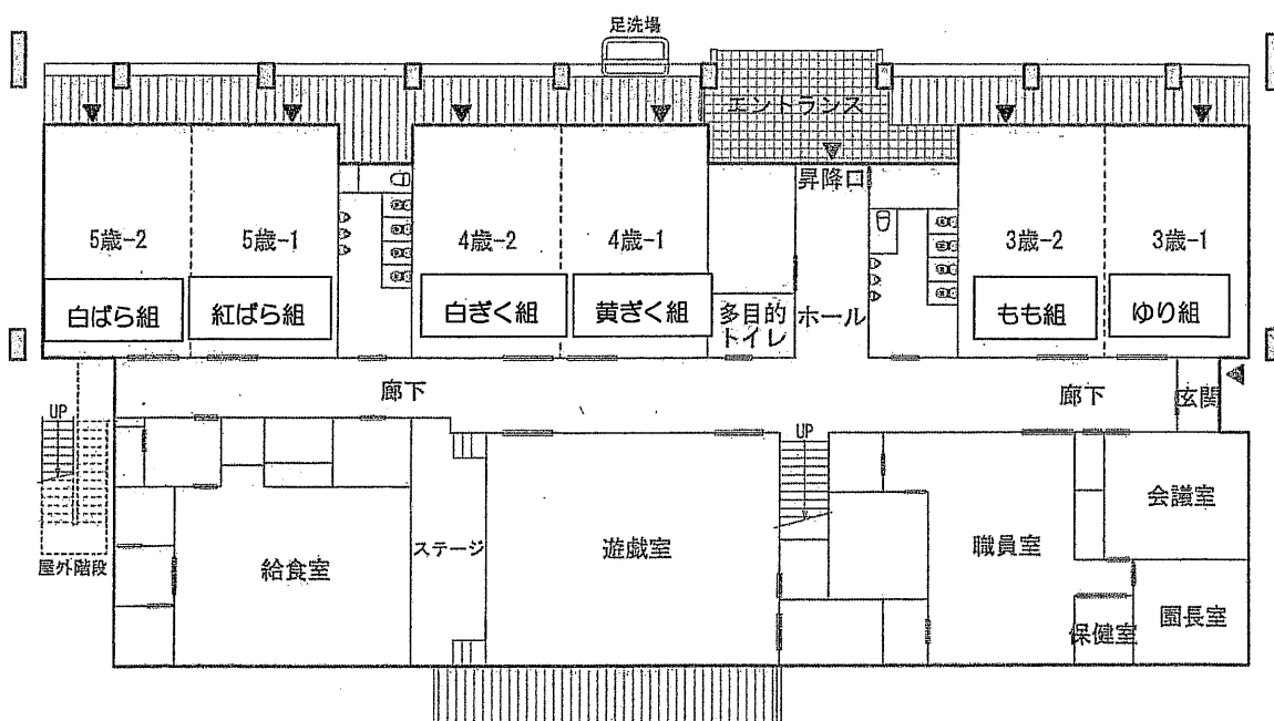
1 階平面図
