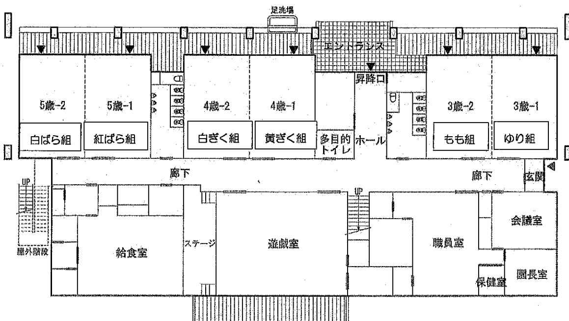
1 階平面図
